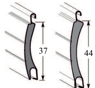
Type 4 Volet roulant maçonnable (intégrée)
